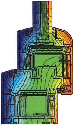
Profieldoorsnede Corona CT 70 Coupe de principe Corona CT 70
